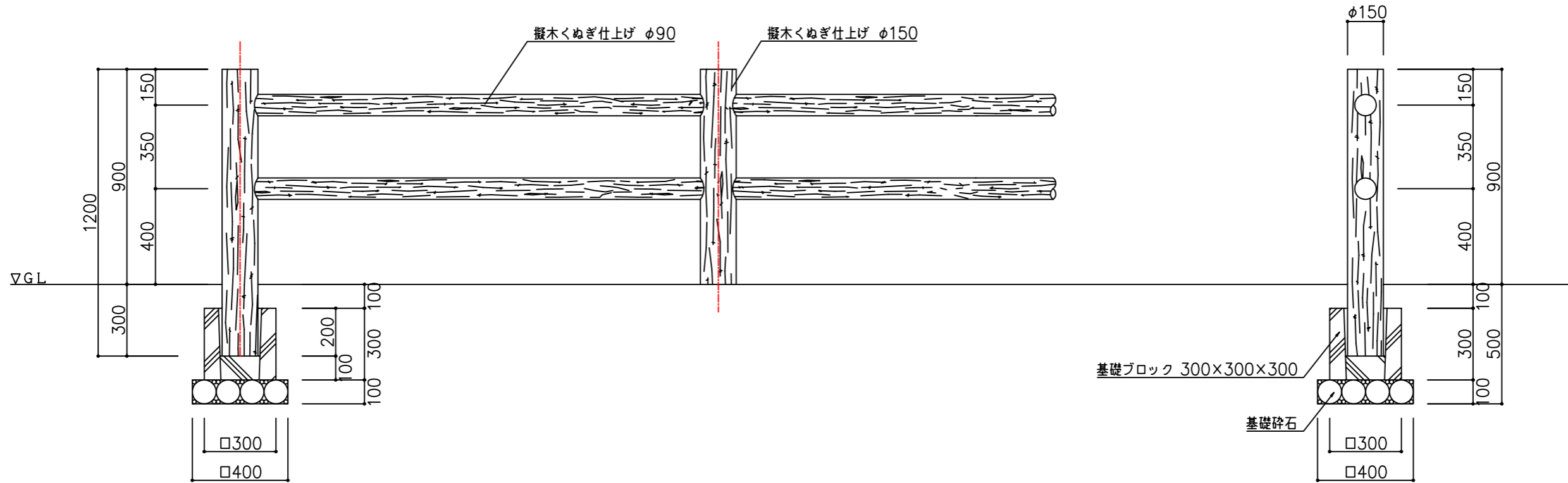
正面図 S=1/20
